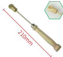
Model: WT01-4 Spur wire embedder
